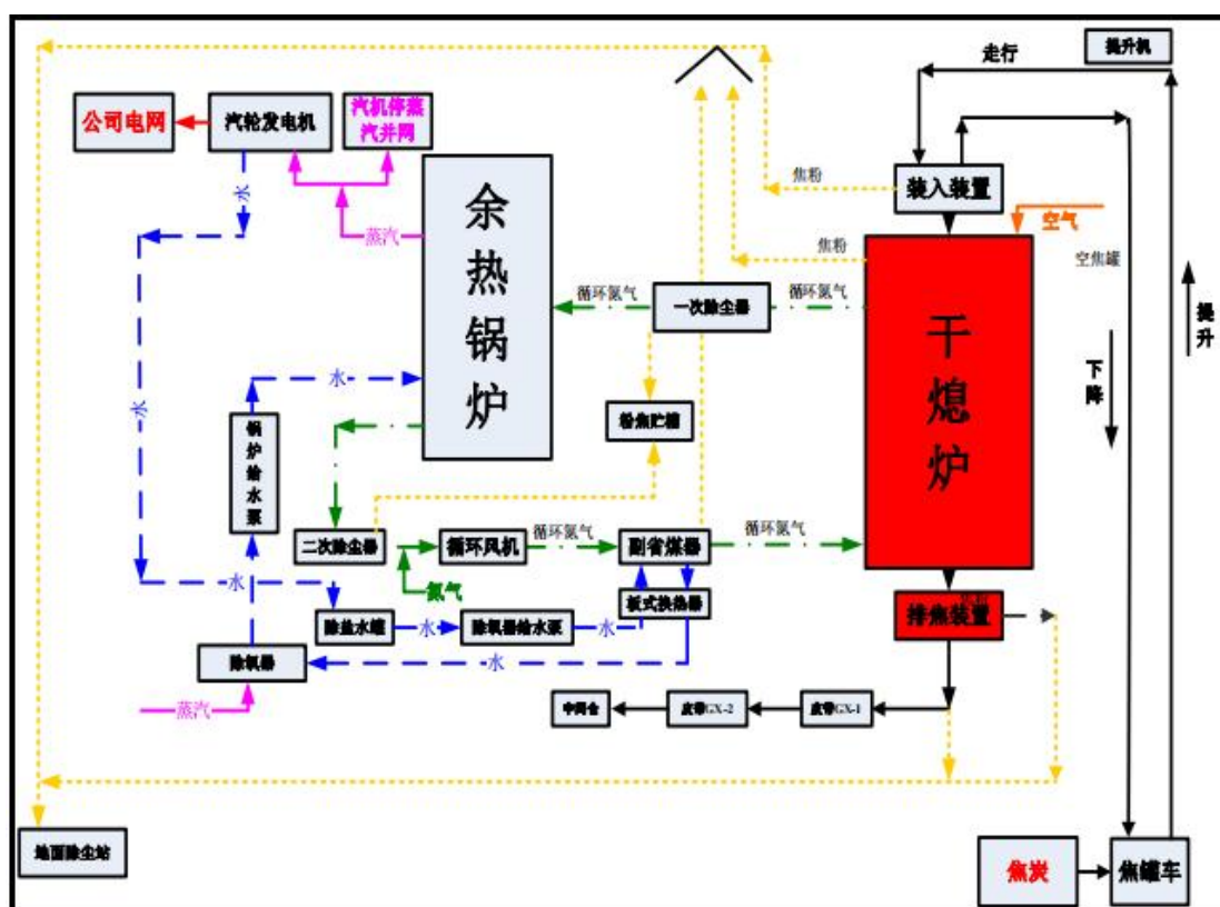
图 3.2-1 干熄焦系统工艺流程图
