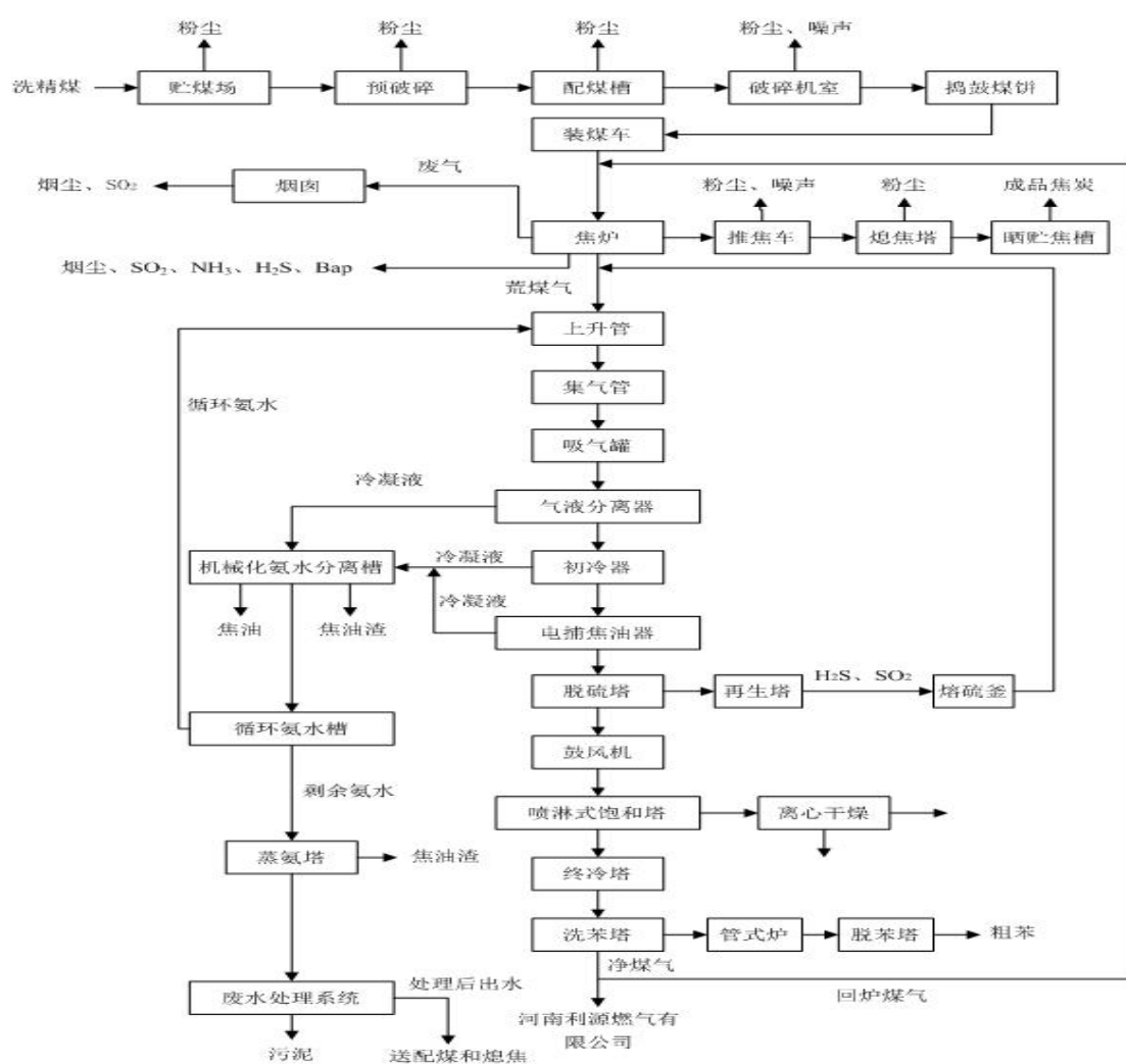
图 3.2-1 生产工艺流程及产排污点环节图
